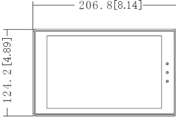
Önden Görünüş
